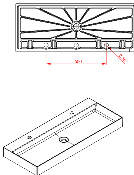
Onderaanzicht
