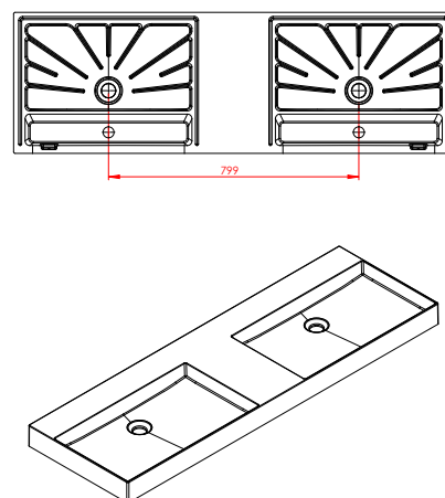
Onderaanzicht
